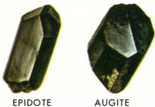
EPIDOTE
