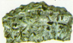
ANDESITE
