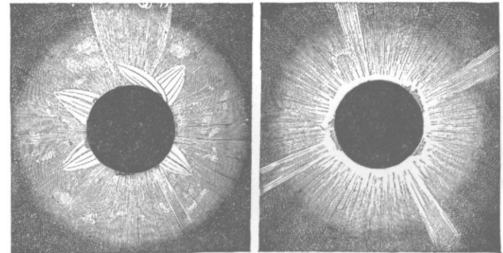
Fig. 155. Eclipse of July 18, 1860, (Feilitzsch).
