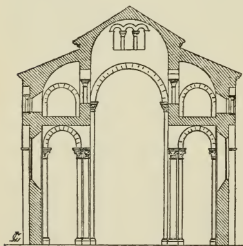
FIG. 97.—SECTION OF NOTRE DAME DU PORT, CLERMONT.
