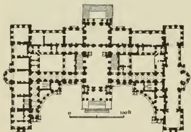
FIG. 188.—PLAN OF BLENHEIM.
