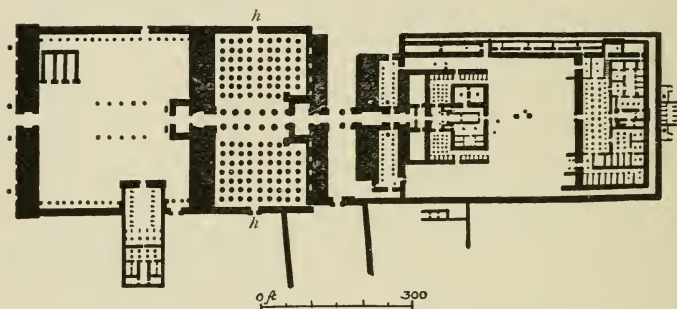
FIG. II.—TEMPLE OF KARNAK. PLAN.
