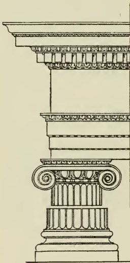
FIG. 43.—ROMAN IONIC ORDER.
