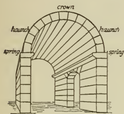
FIG. 46.—BARREL VAULT.
