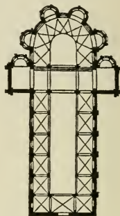
FIG. 96.—PLAN OF NOTRE DAME DU PORT, CLERMONT.
