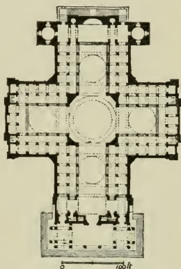
FIG. 202.—PLAN OF PANTHÉON, PARIS.
