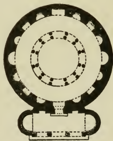
FIG. 66—STA. COSTANZA, ROME.
