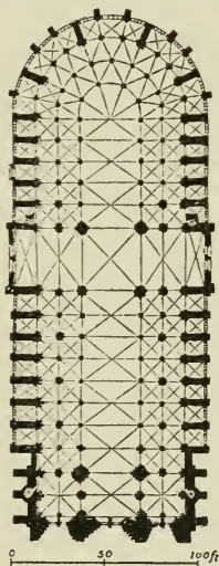
FIG. 116.—PLAN OF NOTRE DAME, PARIS.
