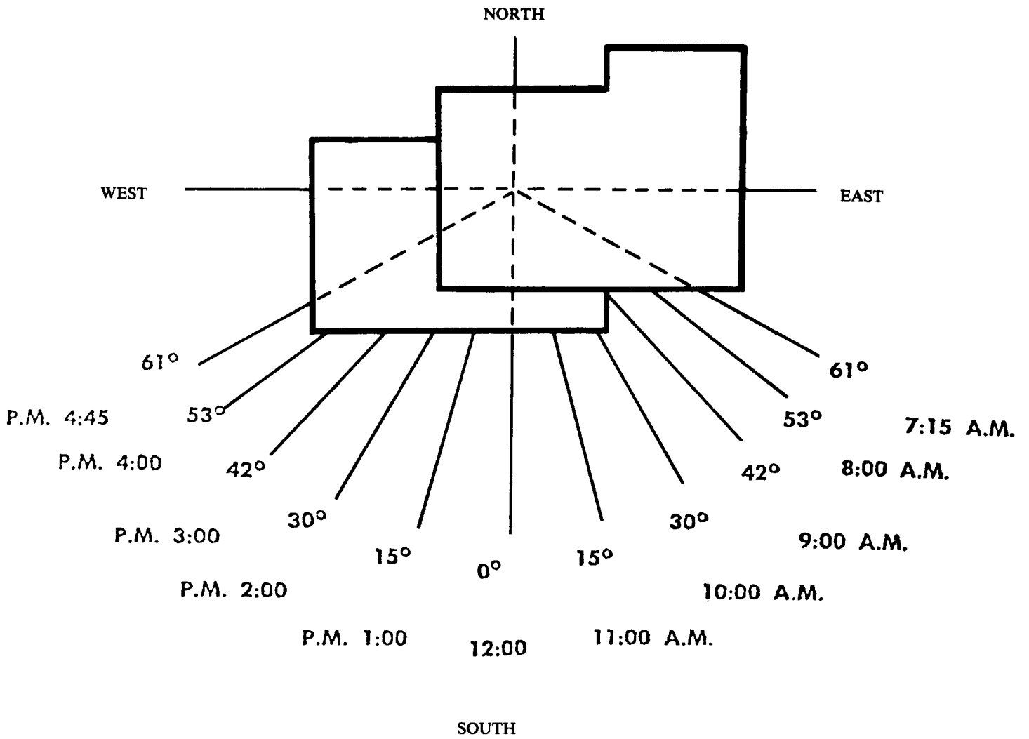
Figure 17. Horizontal angles of the sun December 21; latitude 36°.
