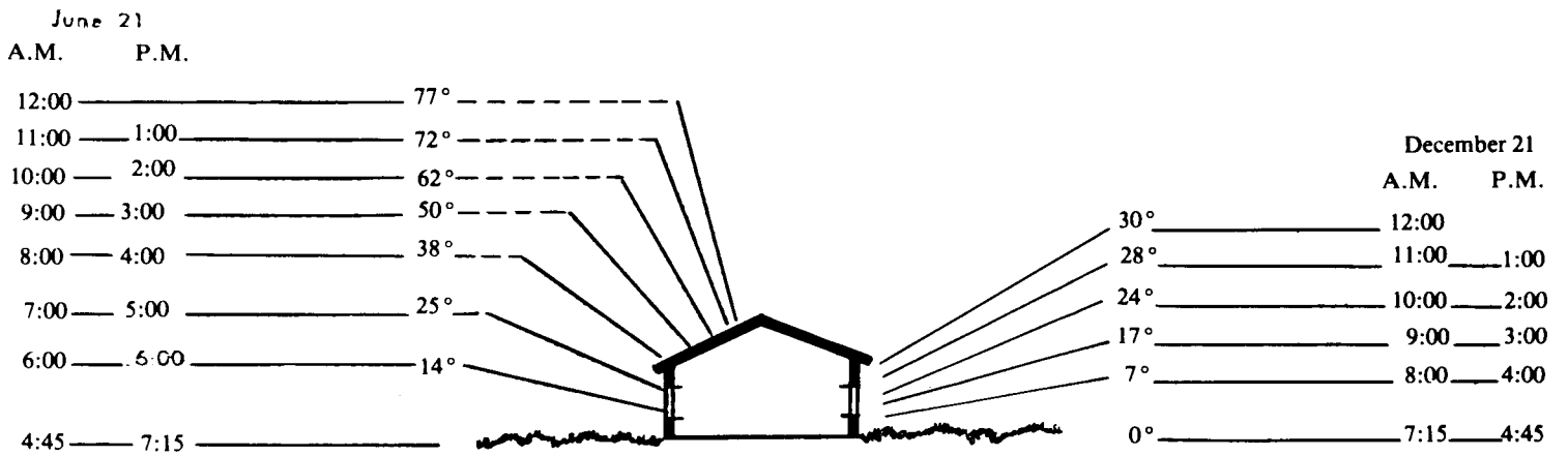
Figure 18. Altitude angles of the sun, latitude 36°.
