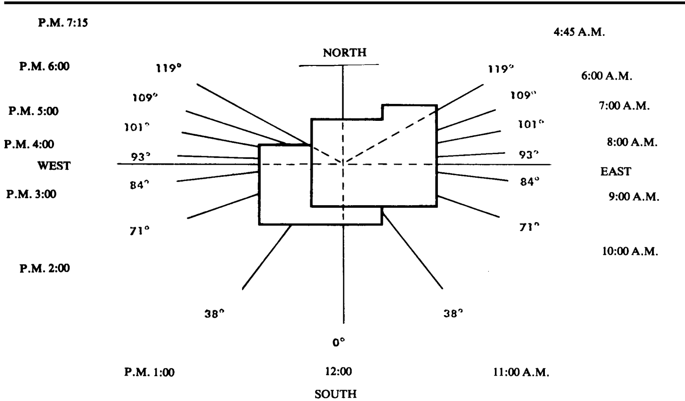
Figure 16. Horizontal angles of the sun July 21; latitude 36^\circ .
