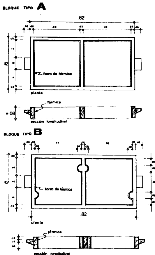
FIGURE 203 : MOULES UTILISÉS À CAYALTI
