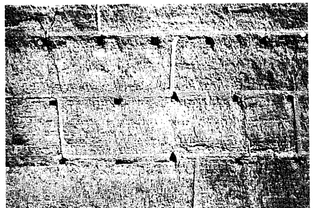
FIGURE 23 : MUR BANCHE AVEC DES JOINTS VERTICAUX (BRESSE)
