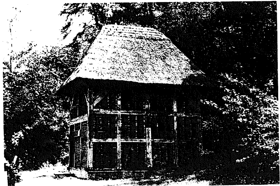
FIGURE 293 : ▶ « CATHERINGTON TREAD WHEEL » XVI e SIECLE (MUSEE EN PLEIN AIR DE SINGLETON) CETTE PETITE MAISON ABRITTE UNE ROUE DANS LAQUELLE MARCHAIT UN HOMME POUR FAIRE REMONTER L'EAU D'UN PUIT. ELLE N'A JAMAIS ETE ENDUITE DE TERRE, CHOSE COURANTE A L'EPOQUE
