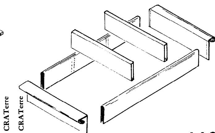
2 - MOULE EN TOLE POUR TROIS BLOCS DE 19 x 39 x 9 cm
