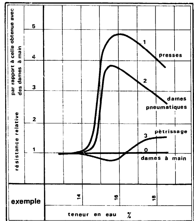
FIGURE 278 : RESISTANCES POUR UNE DEFORMATION DE L'ECHANTILLON DE 5%
