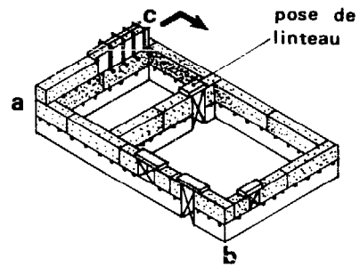
2 ème ASSISE
