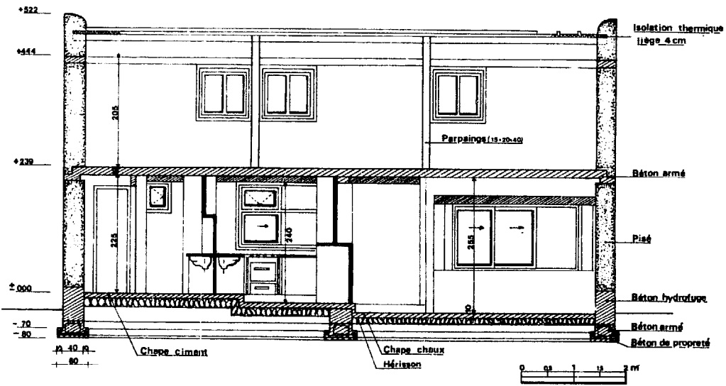
FIGURE 113 : COUPE LONGITUDINALE
