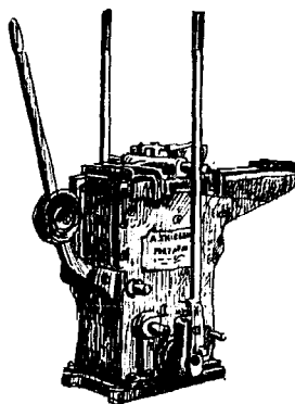
PRESSE PM A BRAS
