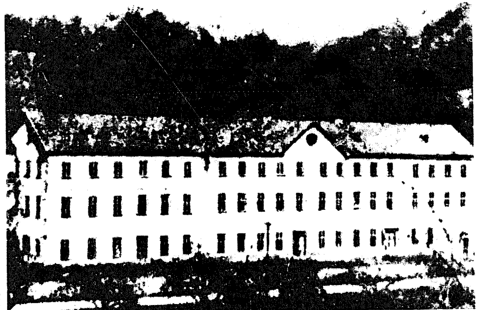
FIGURE 66 : FABRIQUE DE CERAMIQUE (PISE) BATIE PAR WIMPF AU DEBUT DU XIX e SIECLE. APRES 45 ANS D'ABANDON TOTAL (TOIT ET VITRES BRISES), CETTE CONSTRUCTION CONSERVE EN 1920 DES MURS ET DES ENDUITS INTACTS. IL A FALLU DETUIRE A LA DYNAMITE CETTE USINE EN PISE (STABILISE PAR LA CHALEUR DES FOURS) QUI N'EXISTE PLUS DE NOS JOURS.
