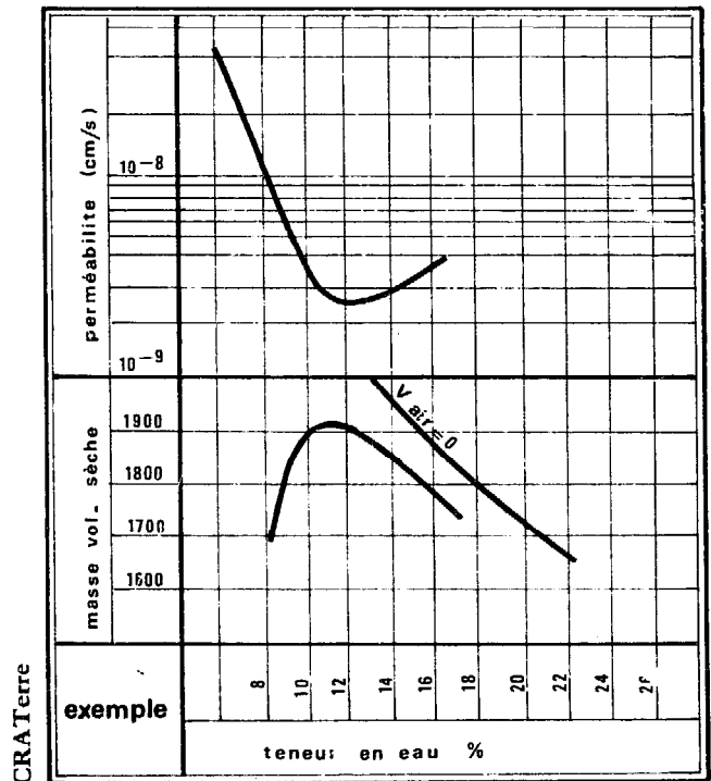
FIGURE 276 : PERMEABILITE ET T.E.O.
