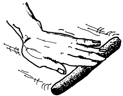
FIGURE 160 : TEST POUR VERIFIER L'APTITUDE DE LA TERRE A LA FABRICATION DE L'ADOBE
