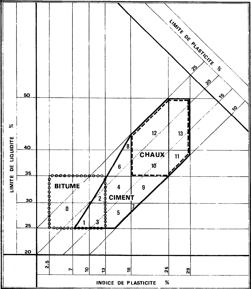
▲ FIGURE 281 : FUSEAU DE STABILISATION POUR LE CIMENT, LA CHAUX, LE BITUME, SEULS LES ELEMENTS FINS (INFERIEURS A 0,5 mm) SONT PRIS EN CONSIDERATION
