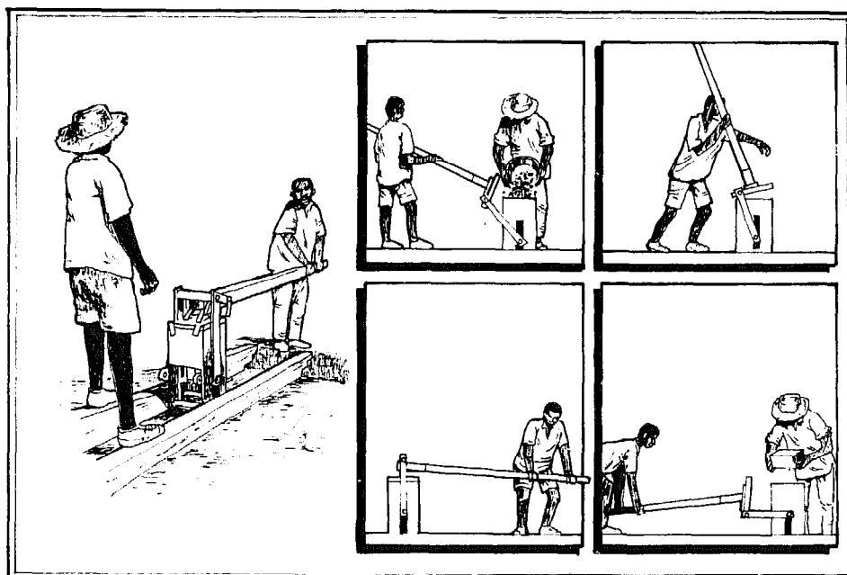
FIGURE 222 : PRESSE TEK-BLOC - REMPLISSAGE DU MOULE - COMPRESSION - DEMOULAGE
