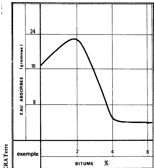
FIGURE 290 : ESSAI D'ABSORPTION
