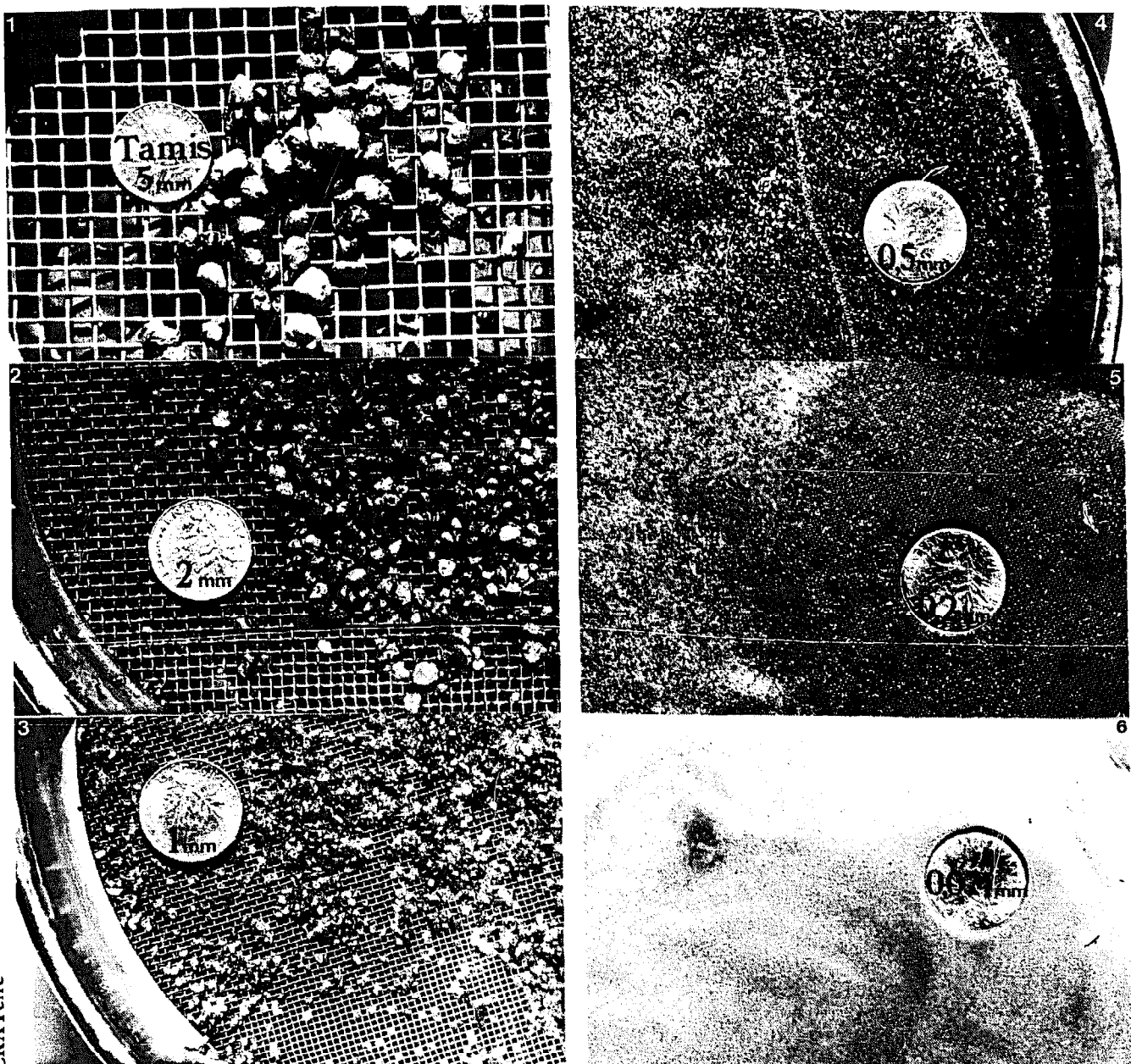
FIGURE 242 : LES REFUS DOIVENT ETRE TRES PROPRES AVANT D'ETRE ETUVES ET PESES
