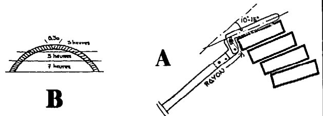
FIGURE 323 : CONSTRUCTION D'UNE COUPOLE SANS CINTRE
