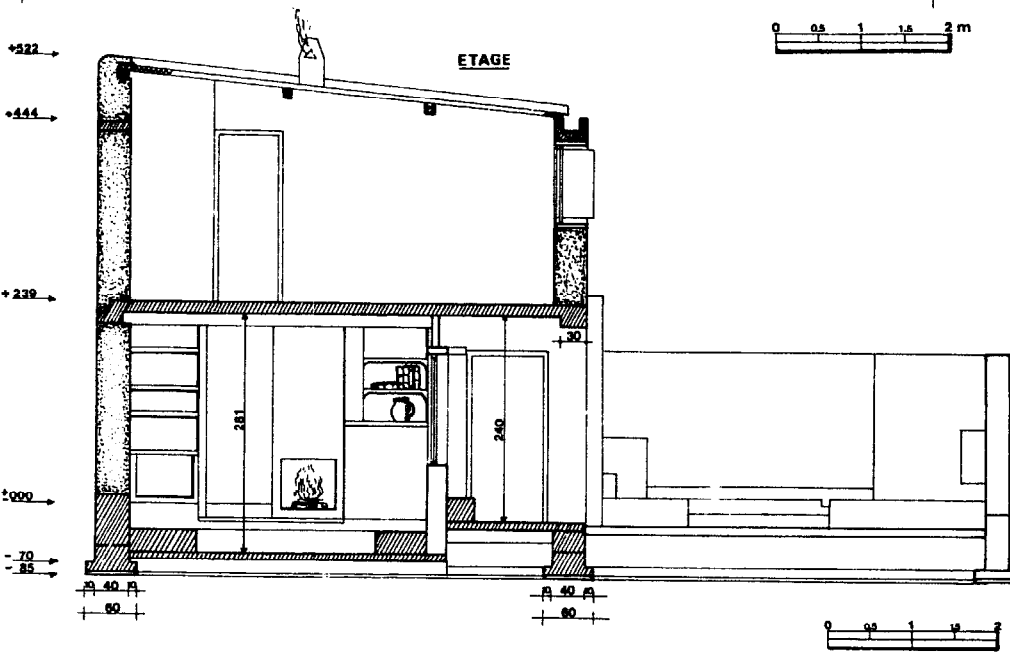
FIGURE 112 : COUPE TRANSVERSALE
