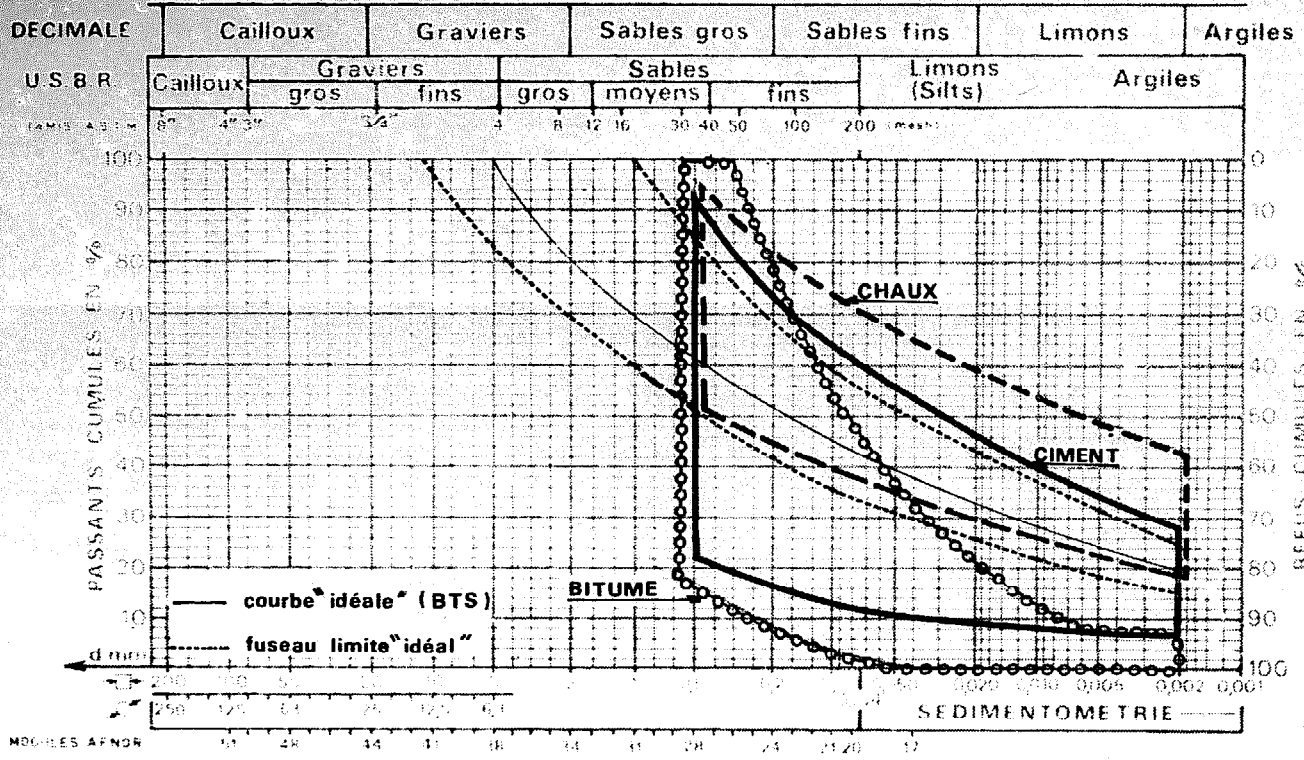
▲ FIGURE 281 : FUSEAU DE STABILISATION POUR LE CIMENT, LA CHAUX, LE BITUME, SEULS LES ELEMENTS FINS (INFERIEURS A 0,5 mm) SONT PRIS EN CONSIDERATION
