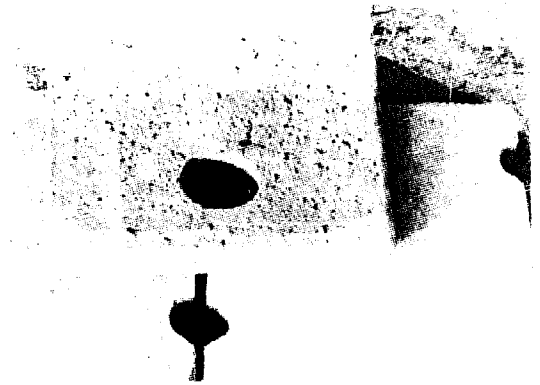
FIGURE 204 : BRIQUES TROUÉES POUR RENFORCEMENT VERTICAL
