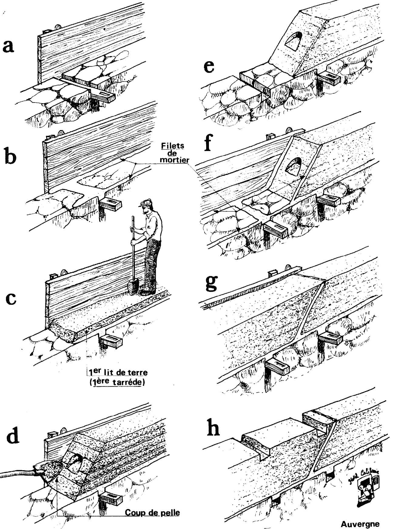
FIGURE 17 : DIFFERENTES PHASES DE LA REALISATION D'UNE BANCHEE
