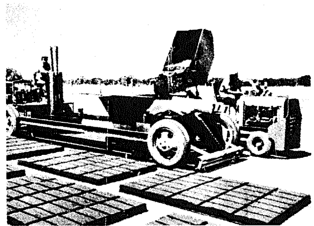
FIGURE 174 : MACHINE A MOULER DE LA « HANS SUMPFF COMPANY » A FRESNO (CALIFORNIE)
