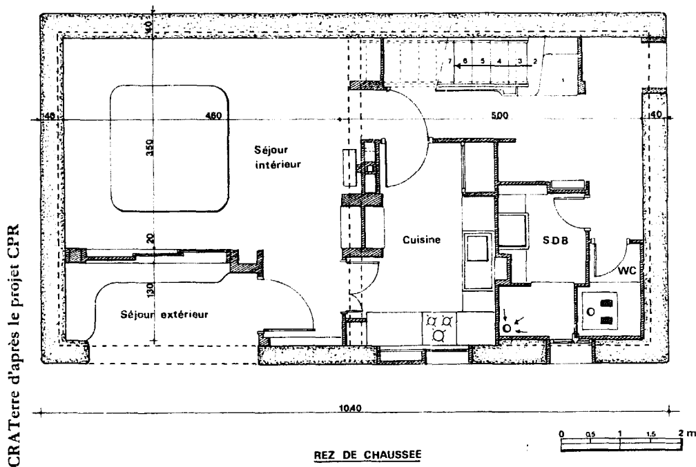
FIGURE 110 : REZ-DE-CHAUSSEE
