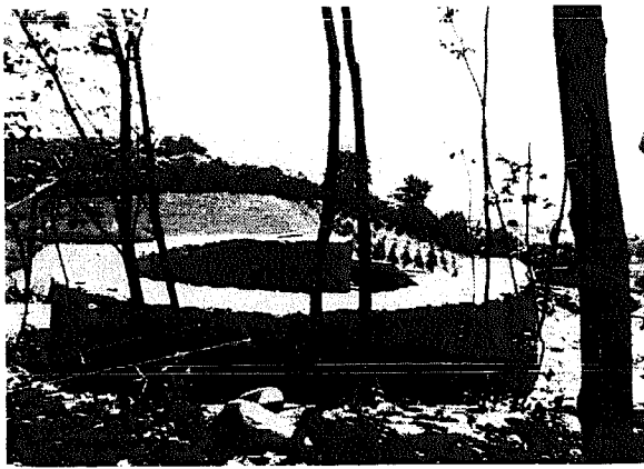
▲ FIGURE 96 : EXPERIENCE DU GROUPE « PALAFITTE » DE L'UP D'ARCHITECTURE DE GRENOBLE EN 1975 AU PIN (ISERE) - CONSTRUCTION CIRCULAIRE EN PISE
