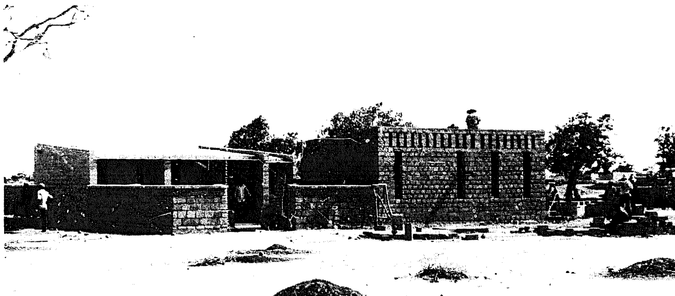
FIGURE 224 : REALISATION EN BRIQUES DE TERRE COMPRESSEES A CISSIN, OUAGADOUGOU (HAUTE-VOLT.A)
