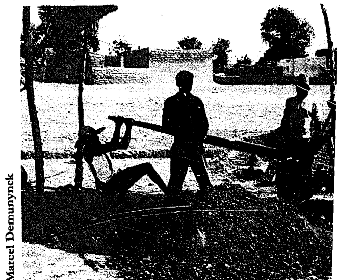
FIGURE 223 : FABRICATION DE BRIQUES AVEC UNE PRESSE TEK BLOC (HAUTE-VOLTA)
