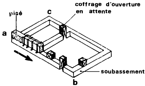
1 ère ASSISE
