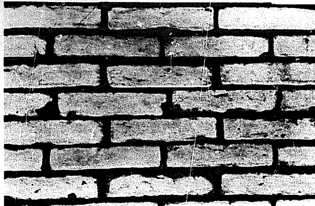
FIGURE 184 : APPAREILLAGE DE BRIQUES STABILISEES, PROJET CAYALTI (PEROU)
