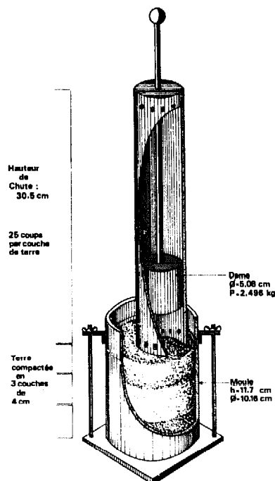
FIGURE 257 : MATERIEL POUR L'ESSAI PROCTOR
