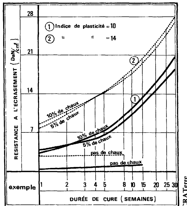
FIGURE 288 : TEMPS DE CURE ET RESISTANCE
