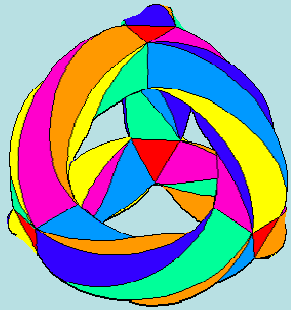
3-torus
