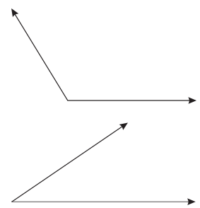
Oblique angle
