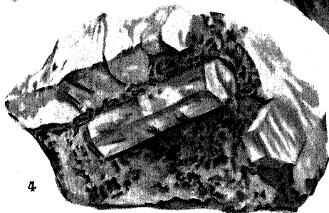
1, Sodalite. 2, Lapis-lazuli. 3, Leucite. 4, Beryl.
