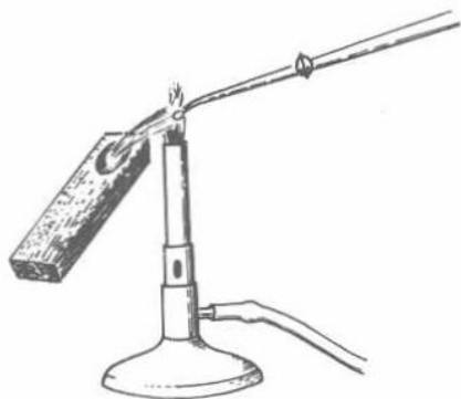
Fig. 4 Charcoal test
