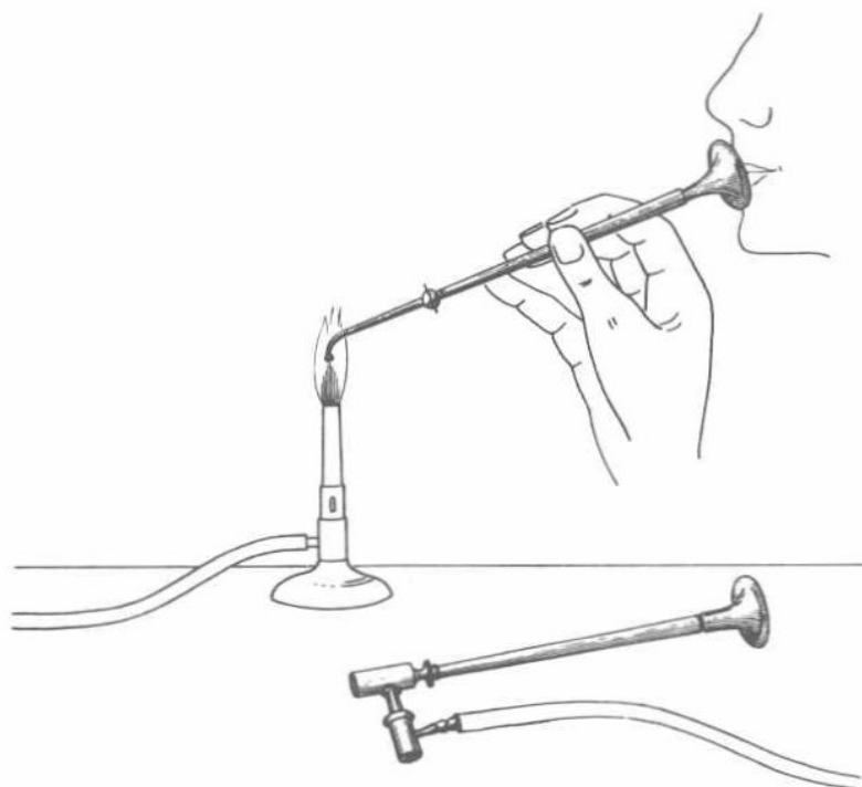
Fig. 3 Blowpipes
