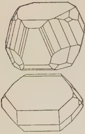
1. Miargyrite (Zacatecas, Mexico)
