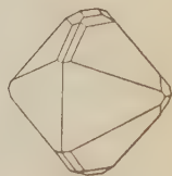
6. Brookite p. 133 (Tremadoc, Wales)
