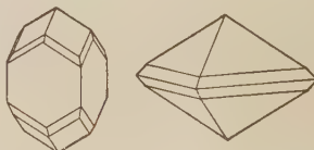
4. Zircon p. 302 (Brudenell, Ontario)
