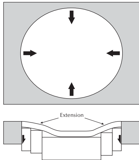
(d) Downsag
