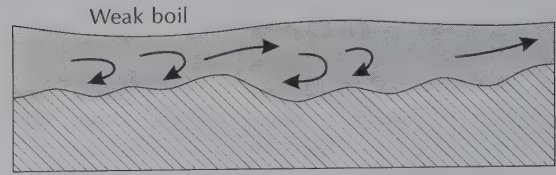
(d) Washed-out dunes ( F \geq 1 )
