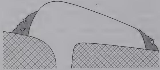
(b) Coulée
