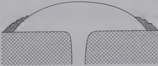
(c) Peléean dome
