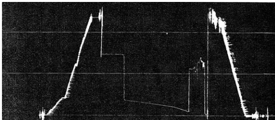
Fig. 4.16 Leaking dual closed—in-pressure valve “DCIPV” (Fuite au Vanne de fermeture et ouverture)
