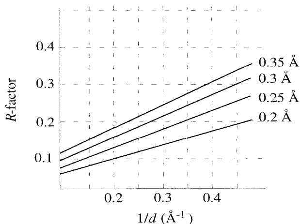
Figure 8.3 Luzzati diagram.
