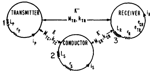
Figure 7.6. Electric-circuit analogy for EM system.
