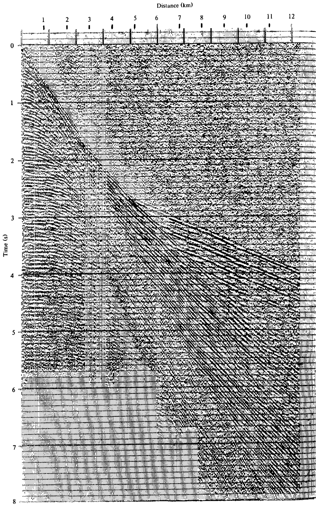
Figure 4.86. Marine refraction profile. (Courtesy Compagnie Générale de Géophysique.)
