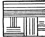
Fig. 82. — Macles de l'albite et de la péricline dans une section de la zone ph^1 .
