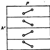
FIG. 118. — Chondrodite maclée. Sections g^1 .
