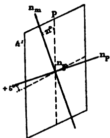
FIG. 78. Orthose non déformée. Section g^1 .
