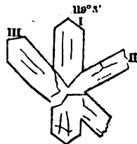
FIG. 157. — Macles en croix de l'hypersthène.
