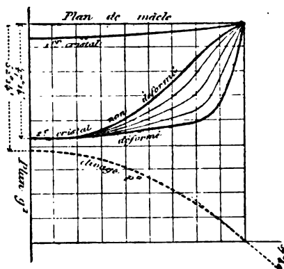
FIG. 9. — Macle de Carlsbad zone pg^1 .
