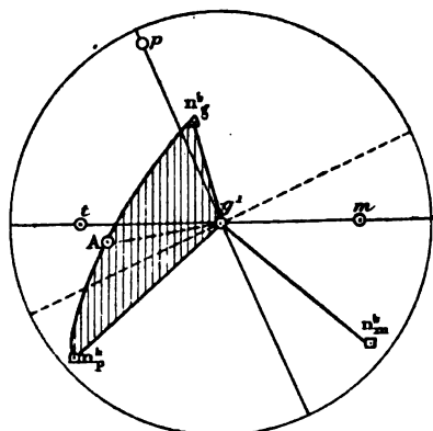
FIG. 100. — Projection sur g^1 .
