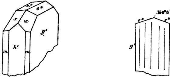
FIG. 155. — Pointements de l'hypersthène. FIG. 156. — Profil de la section h' .
