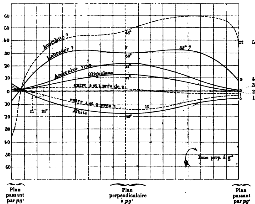
FIG. 89. — Zone perpendiculaire à g' , rapportée à la trace g' , à partir du plan passant par pg' , dans le sens des aiguilles d'une montre.
