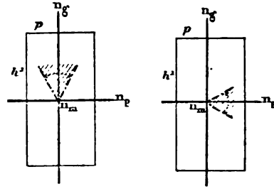
Enstatite. Hypersthène. FIG. 159. — Sections g' .
