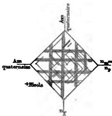
Fig. 126. — Leucite du premier mode. Sections p [h' ou g' ].
