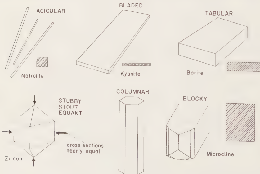
CRYSTAL HABITS
