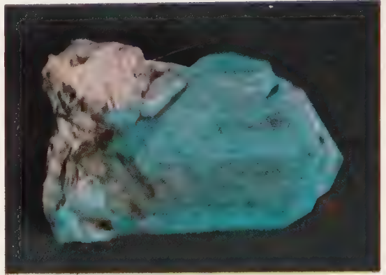
Microcline Feldspar
