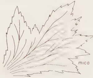
PLUMOSE
