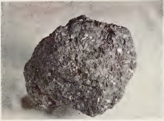
Magnetite
