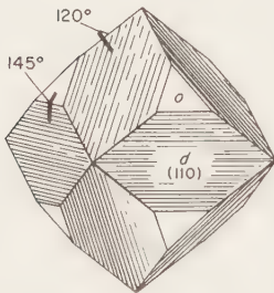
MAGNETITE
