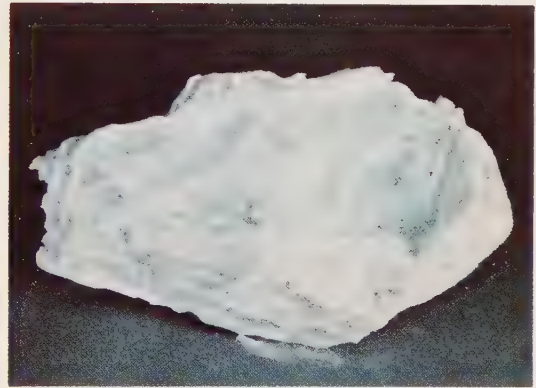
Talc
