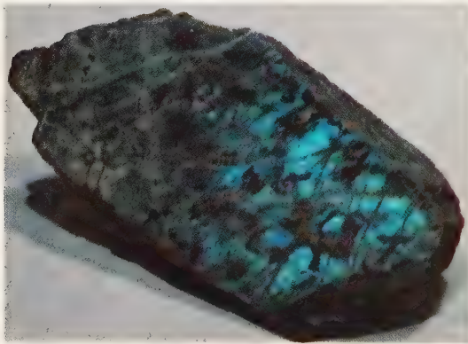
Labradorite Feldspar
