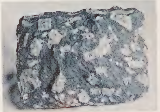
Dolerite Porphyry
