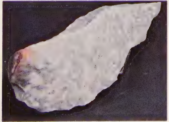
Quartzite
