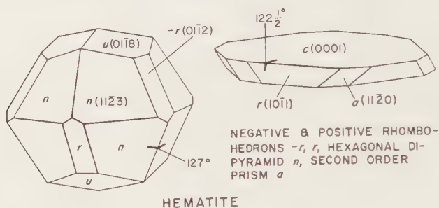
HEMATITE
