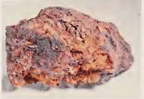
Limonite
