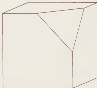
GALENA
