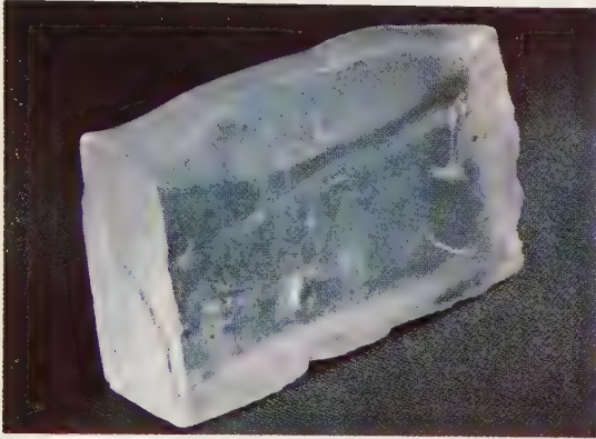
Halite (Salt)
