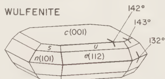
WULFENITE
