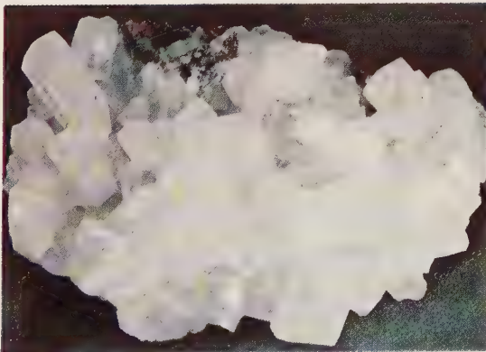
Calcite Crystals
