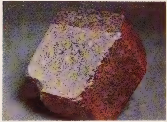
Garnet
