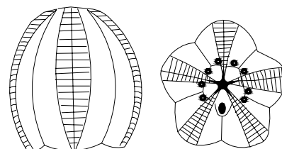
mesoblastus
