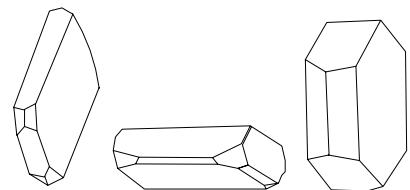
tabular crystals
