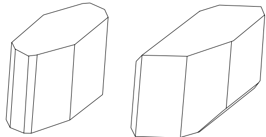
chalcantite crystals
