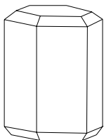
mimetite crystal
