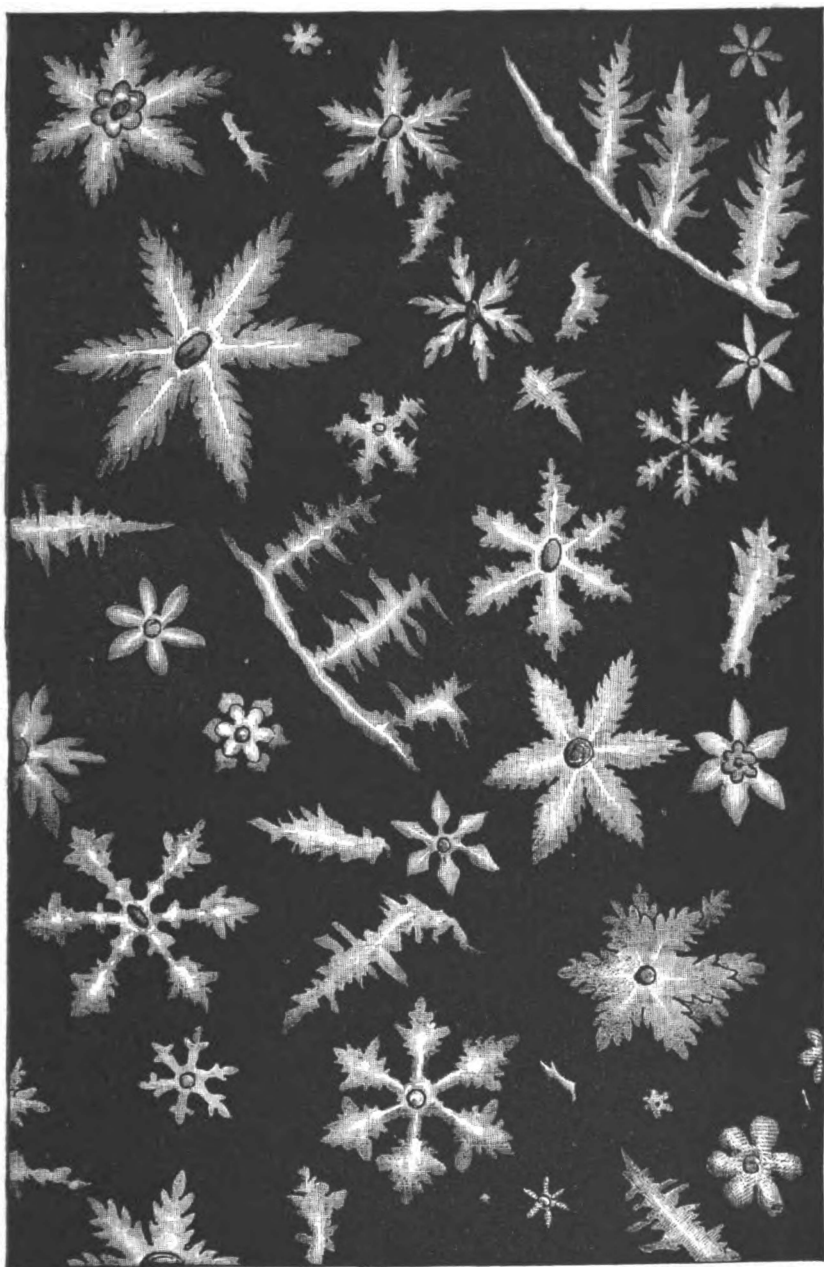
Fig. 1. — Fleurs de la glace d'après M. Tyndall.
