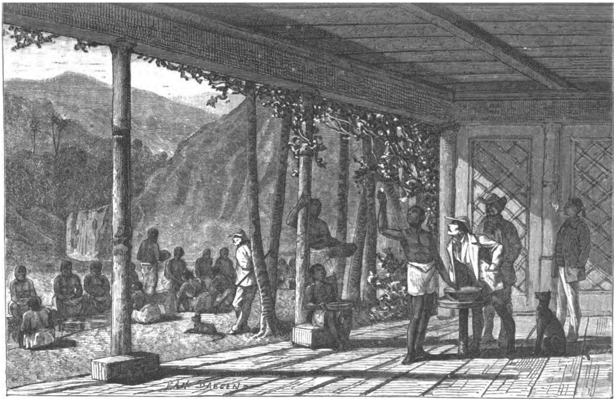
Fig. 13. — Recherche du diamant après le lavage du cascalho.
