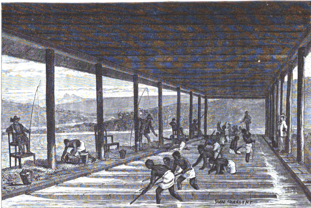
Fig. 12. — Le lavage du cascalho.
