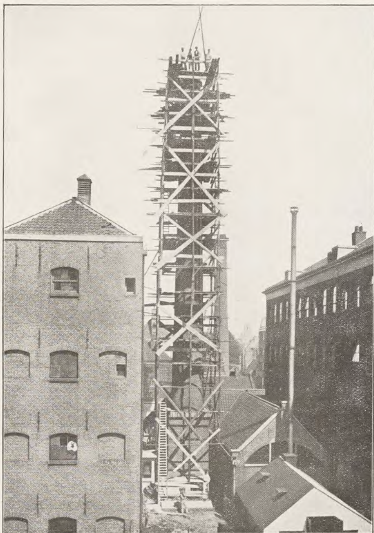
Het repareren van de fabrieksschoorsteen aan de Nieuwe Achtergracht (1885).
