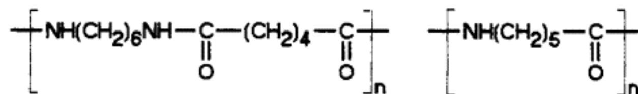
nylon 6,6
