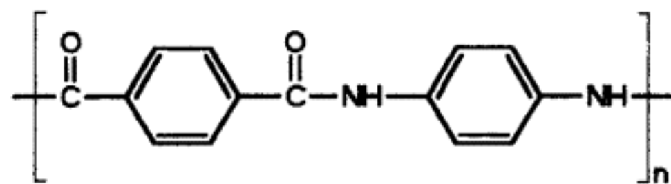
Kevlar
