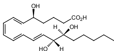
Lipoxin B
