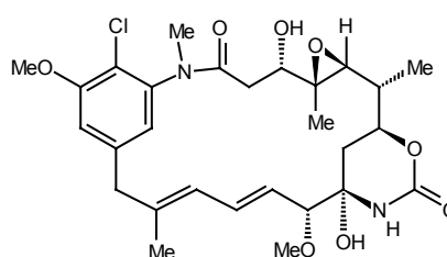
Maytansinol
