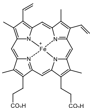
Hemin (Fischer, 1929)
