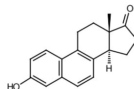
Equilenin (Bachmann, 1939)
