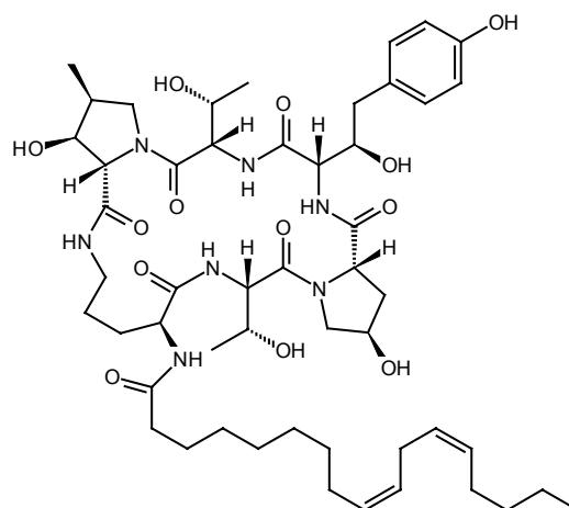
Echinocandin D
