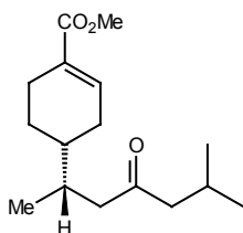
dl-erythro-Juvabione
