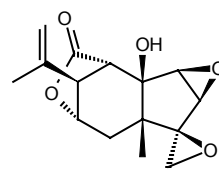
Coriamyrtin
