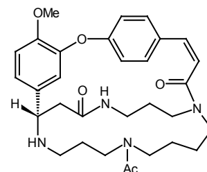
Chaenorhine
