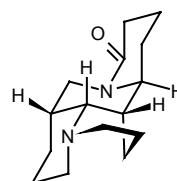
Matrine
