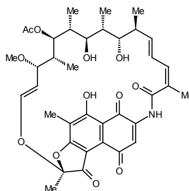
(+)-Rifamycin S
