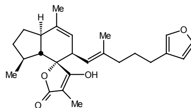
Ircinianin
