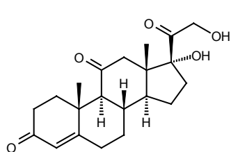
Cortisone
