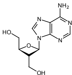
(-)-Oxetanocin
