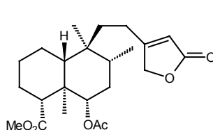
Ajugarin IV
