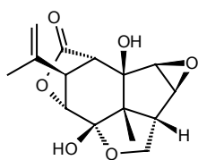
(+)-Asteromurin A
