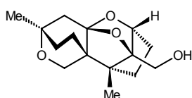
Neosporol
