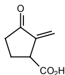
Sarkomycin
