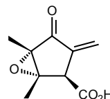
Methyleneomycin A
