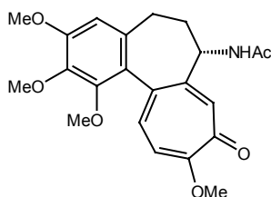
Colchicine (Eschenmoser, 1959)
