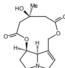
(+)-Dicrotaline
