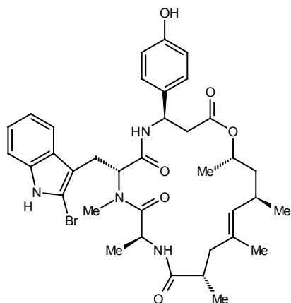
(+)-Jasplakinolide
