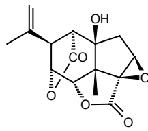
Picrotoxinin
