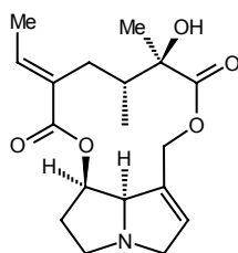
Integerrimine
