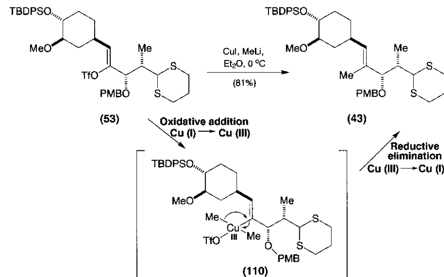
Scheme 17.30.
