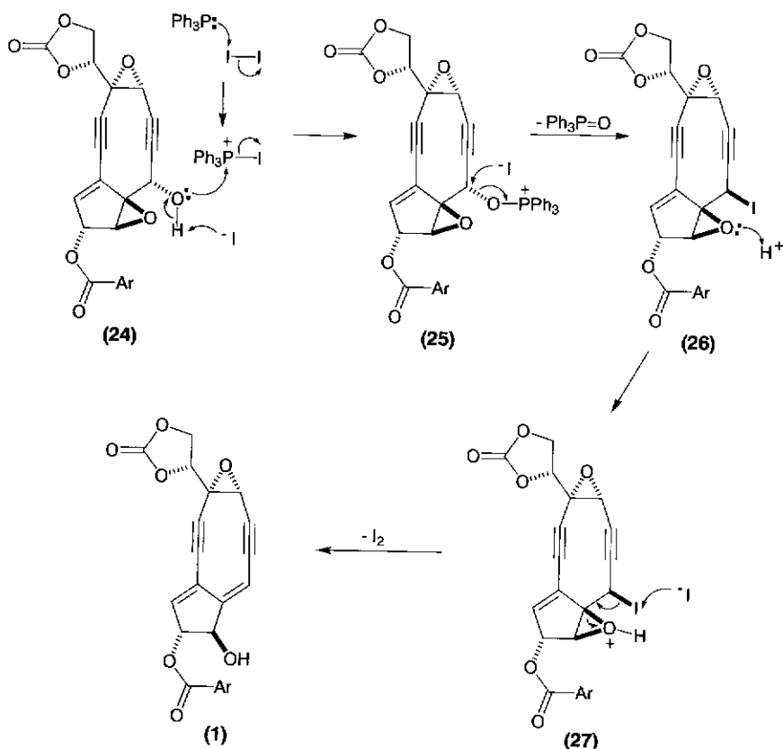
Scheme 8.12.
