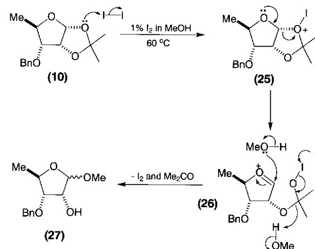
Scheme 12.8.
