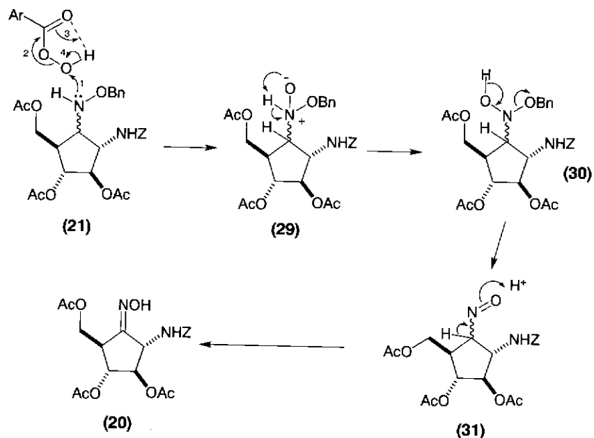
Scheme 11.10.
