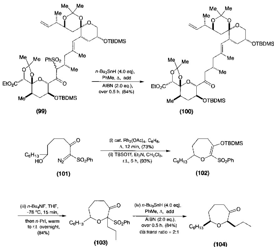
Scheme 17.27.
