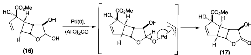
Scheme 6.10.
