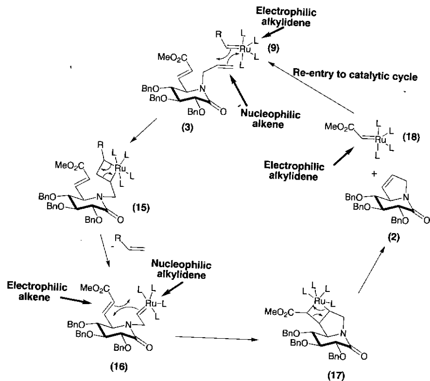
Scheme 9.4.
