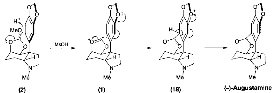
Scheme 16.5.
