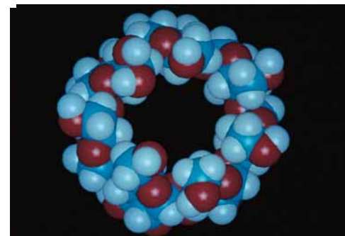
Cycloheptaamylose
