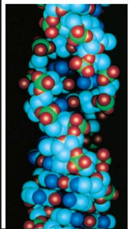
Z DNA
