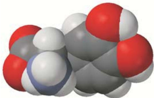
3. Van der Waals model
