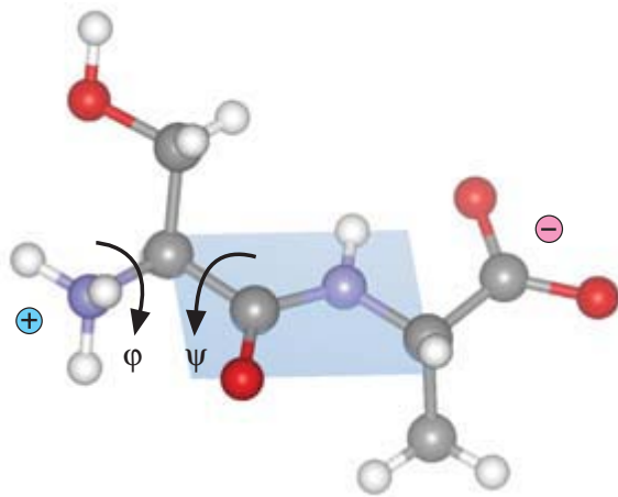
Seryl alanine (Ser-Ala, \text{H}_3\text{N}^+\text{-Ser-Ala-COO}^- , SA)
