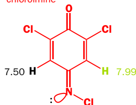
chloroimine
