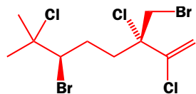
halomon
