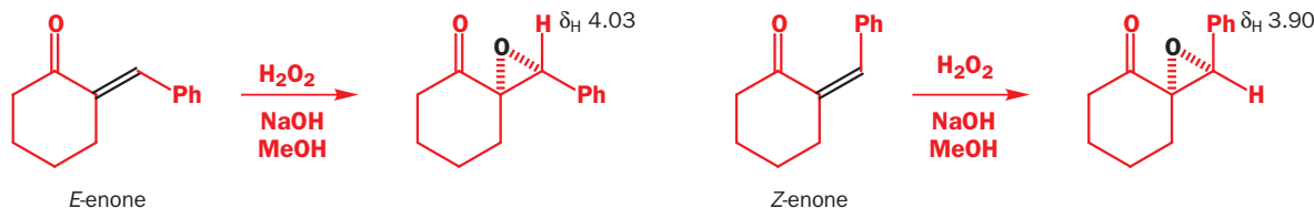
E -enone
