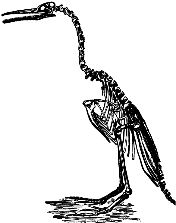
FIG. 3.— HESPERORNIS REGALIS (Marsh).
