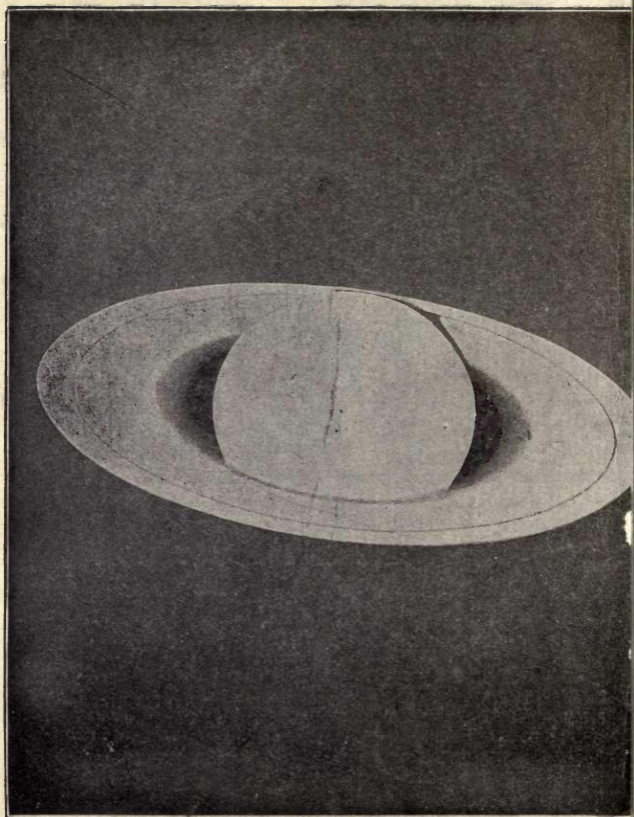
FIG. 1.—THE PLANET SATURN.
