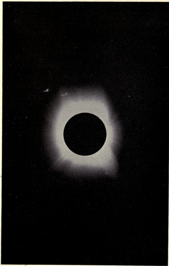
Solar Corona. Total Eclipse.
