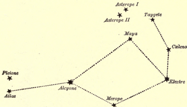
FIG. 25.—The Pleiades.
