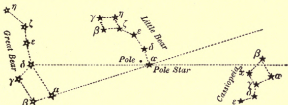
FIG. 5.—To find Cassiopeia.
