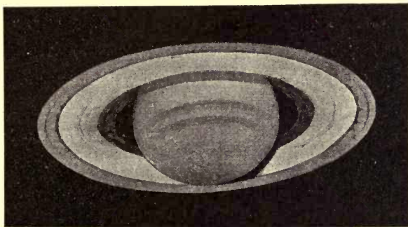
FIG. 47.—Saturn.
