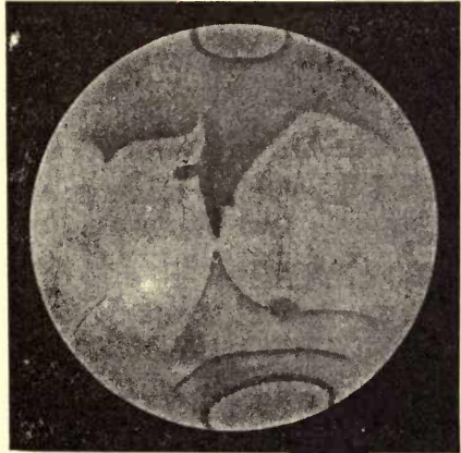
FIG. 41.—Telescopic aspect of the planet Mars (Feb., 1901).
