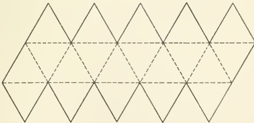
ICOSAHEDRON.
