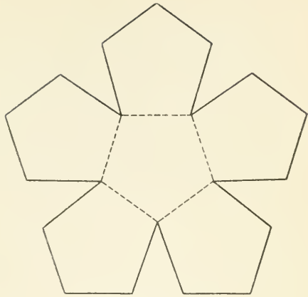
DODECAHEDRON.
