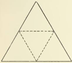
TETRAHEDRON.
