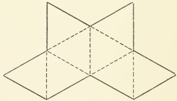
OCTAHEDRON.
