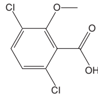
Dicamba [1918-00-9]
