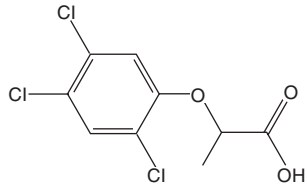
Dicamba [1918-00-9]
