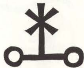
Orpiment
