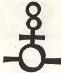
Precipitate
