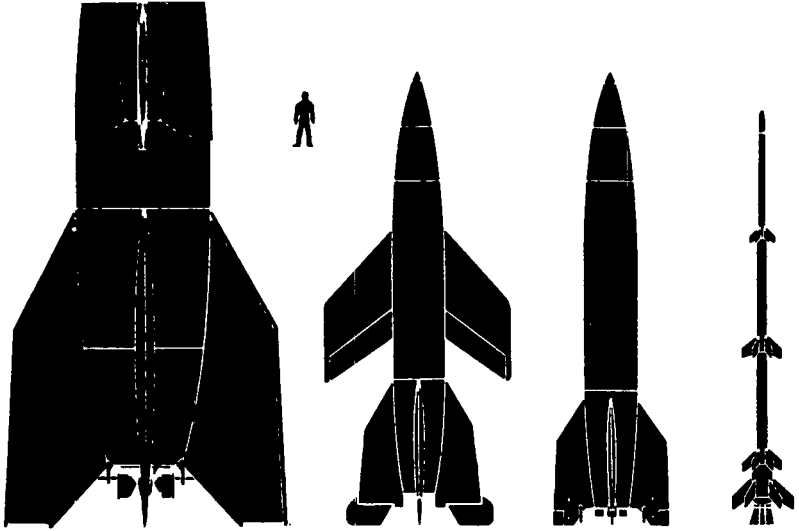
Abb. 217-220. Fernraketen. Von links nach rechts: A-9/A-10; A-4b und A-4 (V 2) von Peenemünde; ganz rechts: Rheinmetall „Rheinbote“.
