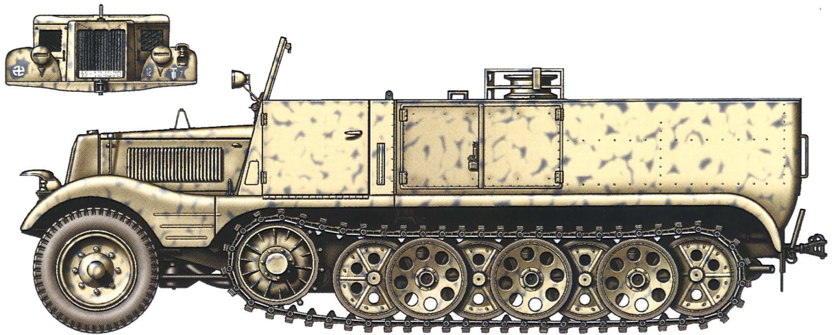
Sd Kfz 11 3to Zgkw z 5. Pułku Artylerii Zmotoryzowanej SS 5. Dywizji Grenadierów Pancernych SS „Wiking”, Kowel, kwiecień 1944 roku. Sd Kfz 11 3to Zgkw tractor from the 5th SS-Artillerie Regiment (motorisiert) 5th SS-Panzer Grenadier Division “Wiking”, Kowel, April 1944.
