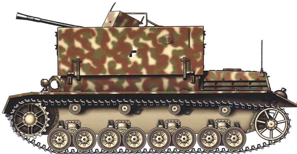
Flakpanzer IV „Möbelwagen” z 9. Dywizjonu Przeciwlotniczego SS, 9. Dywizji Pancerniej SS „Hohenstaufen”, Arnhem, wrzesień 1944 roku. Flakpanzer IV “Möbelwagen” AA tank from the 9th SS-Flak Abteilung 9th SS-Panzer Division “Hohenstaufen”, Arnhem, Holland, September 1944.
