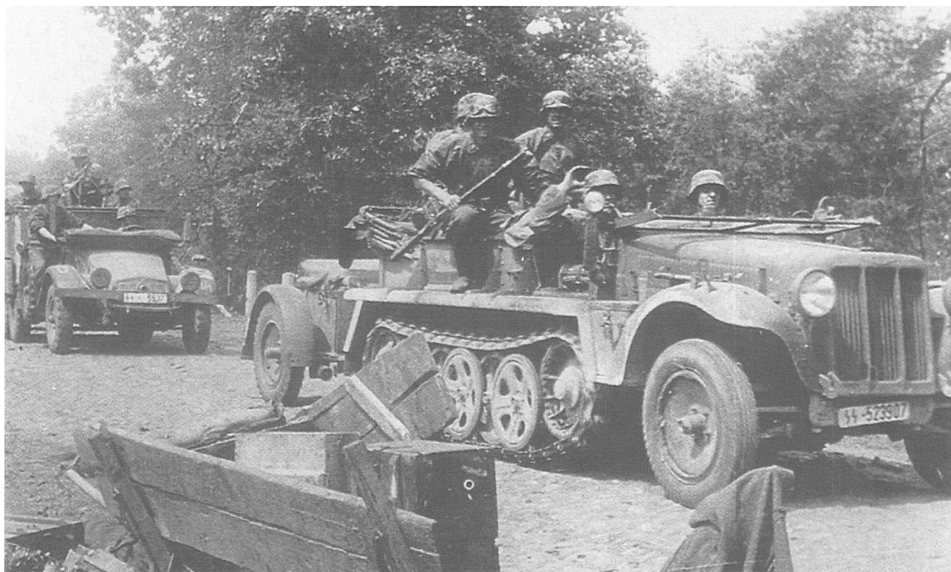
Sd Kfz 10 i Kfz 69 z przyczepami prawdopodobnie z jednostki artylerii 10. Dywizji Pancerniej SS „Fründsberg”, Galicja, wiosna 1944 roku. A Sd Kfz 10 and Kfz 69 with trailers from the artillery unit from the 10th SS-Panzer Division “Fründsberg”, Eastern Front, Spring 1944. [Rolf Michaelis Verlag]
