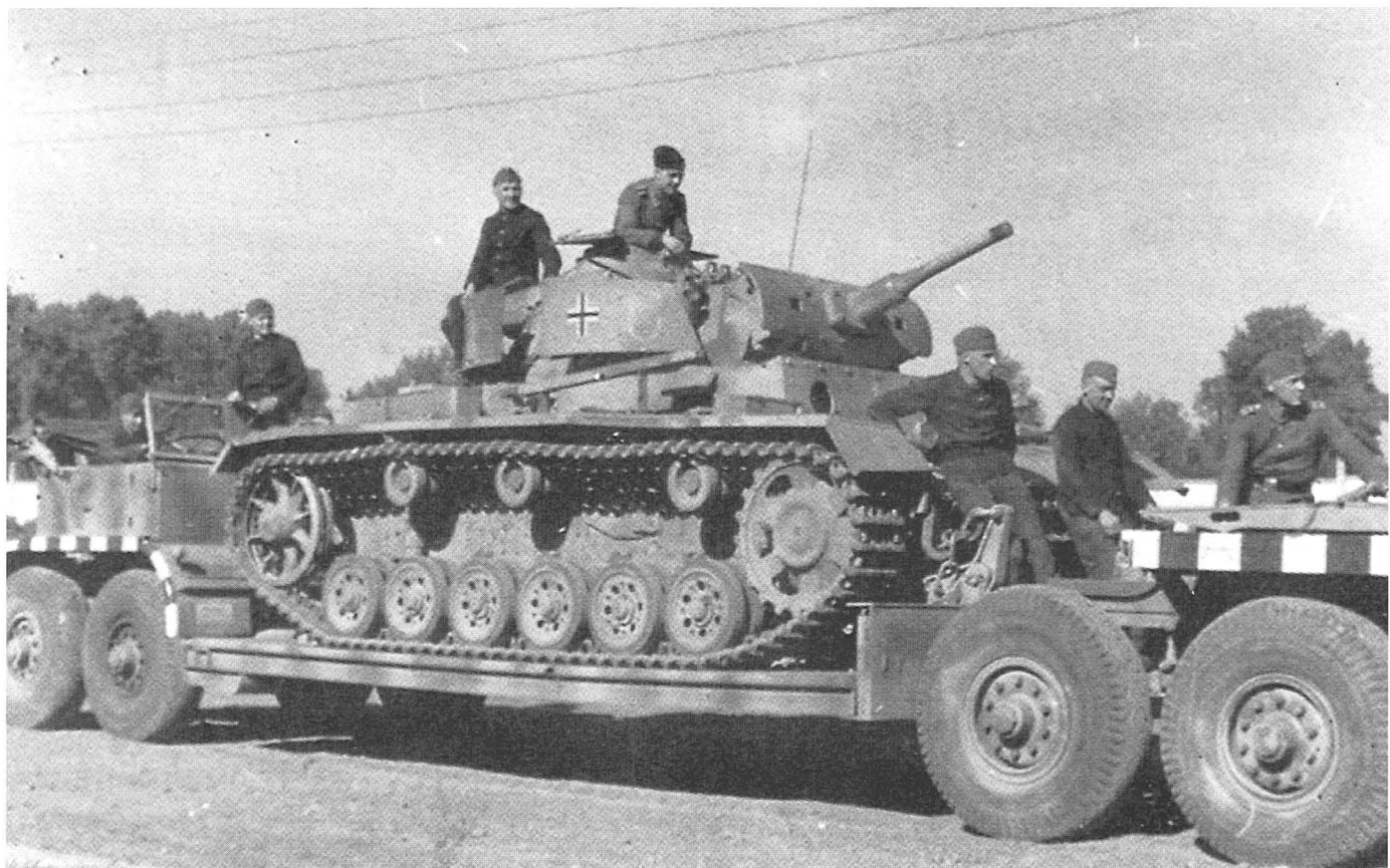
Wóz dowodzenia Panzerbefehlswagen mit 5 cm KwK 39 L/42 oznaczony „C” z 10. Pułku Artylerii Pancerniej SS na naczepie Sd Anh 116, Francja, lato 1943 roku. A Panzerbefehlswagen mit 5 cm KwK 39 L/42 coded “C” command vehicle from the 10th SS-Panzer Artillerie Regiment on Sd Anh 116 trailer in France, Summer 1943. [Rolf Michaelis Verlag]
