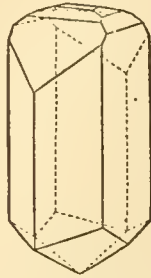
FIG. 2.—Electric Calamine.
