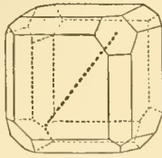
FIG. 3.—Boracite.
