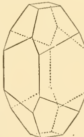
FIG. 6.—Fergusonite.
