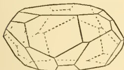
FIG. 4.—Ilmenite.
