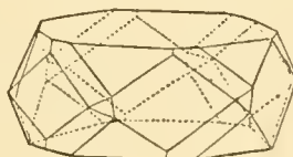
FIG. 5.—Apatite.
