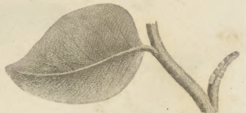
Fig. 25. Coccus.
