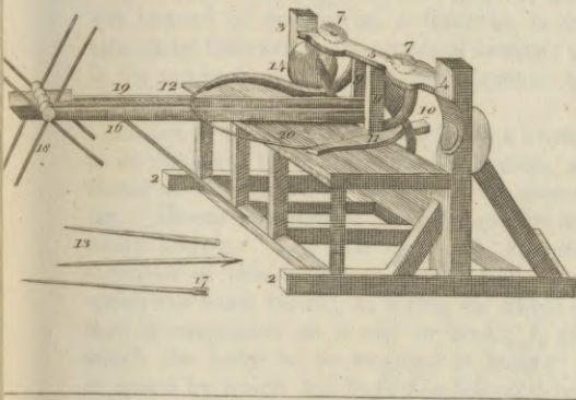
BALISTA. Fig. 6.
