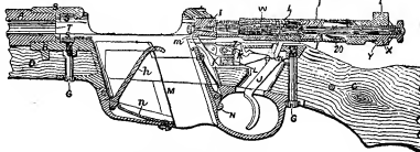
FIG. 13.—Mannlicher, 1895.
