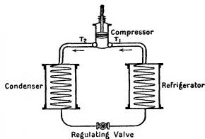
FIG. 2.—Vapour Compression Machine.
