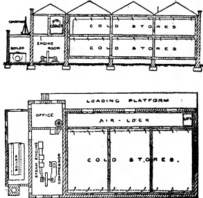
FIG. 7.—Cold Stores.
