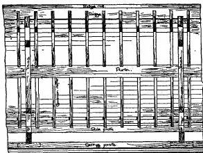
Sectional elevation on AA.
