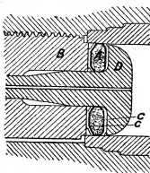
FIG. 52.—De Bange Obturator.
