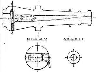
FIG. 8.—Cavalli Gun, 1845.
