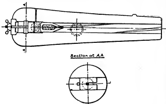
FIG. 9.—Wahrendorff Gun, 1846.
