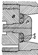
FIG. 53.—Steep Cone de Bange Obturator.
