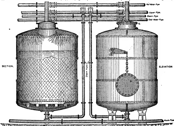
FIG. 3.—Sinclair Esparto Boiler.
