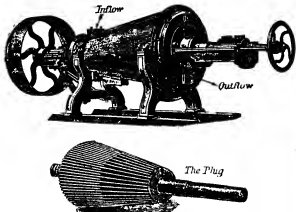
FIG. 9.—Jordan Beater.
