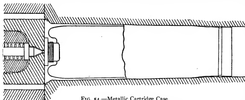
FIG. 54.—Metallic Cartridge Case.
