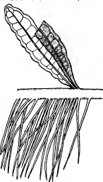
FIG. 2.— Choffatia Francheti .
