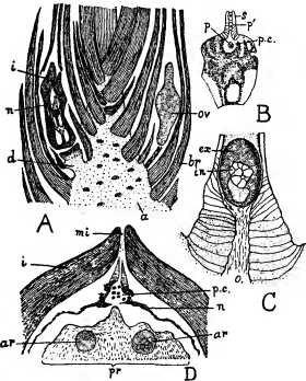
FIG. 32.— Cordaitanthus .
