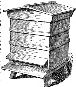
FIG. 16.—Exterior, W.B.C. Hive.
