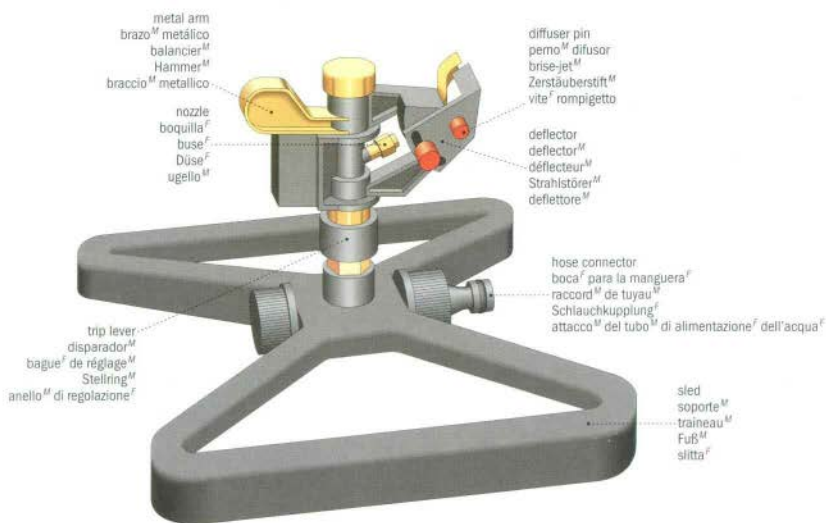
impulse sprinkler irrigador M de impulso M arroseur M canon M Impulsregner M irrigatore M a impulsi M
