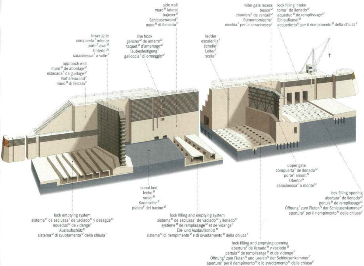
canal lock: side view esclusa f : vista f lateral écluse f : vue f latérale Schleuse f : Seitenansicht f chiusa f di un canale M : vista f laterale
