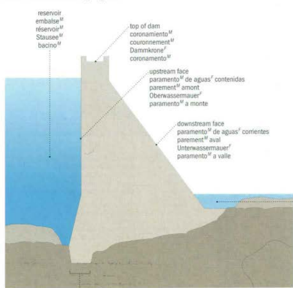
cross section of a gravity dam sección transversal de una presa de gravedad coupe d'un barrage poids Schwergewichtstaudamm im Querschnitt sezione trasversale di una diga a gravità
