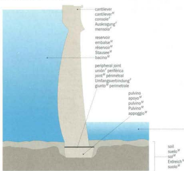
cross section of an arch dam sección transversal de una presa de bóveda coupe d'un barrage voûte Bogenstaudamm im Querschnitt sezione trasversale di una diga a volta
