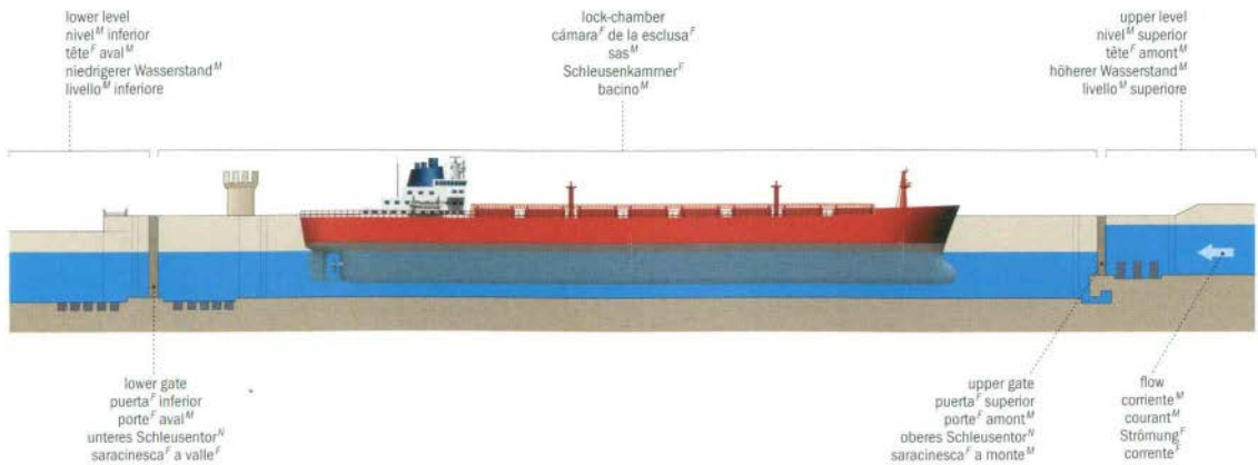
canal lock: side view esclusa f : vista f lateral écluse f : vue f latérale Schleuse f : Seitenansicht f chiusa f di un canale M : vista f laterale
