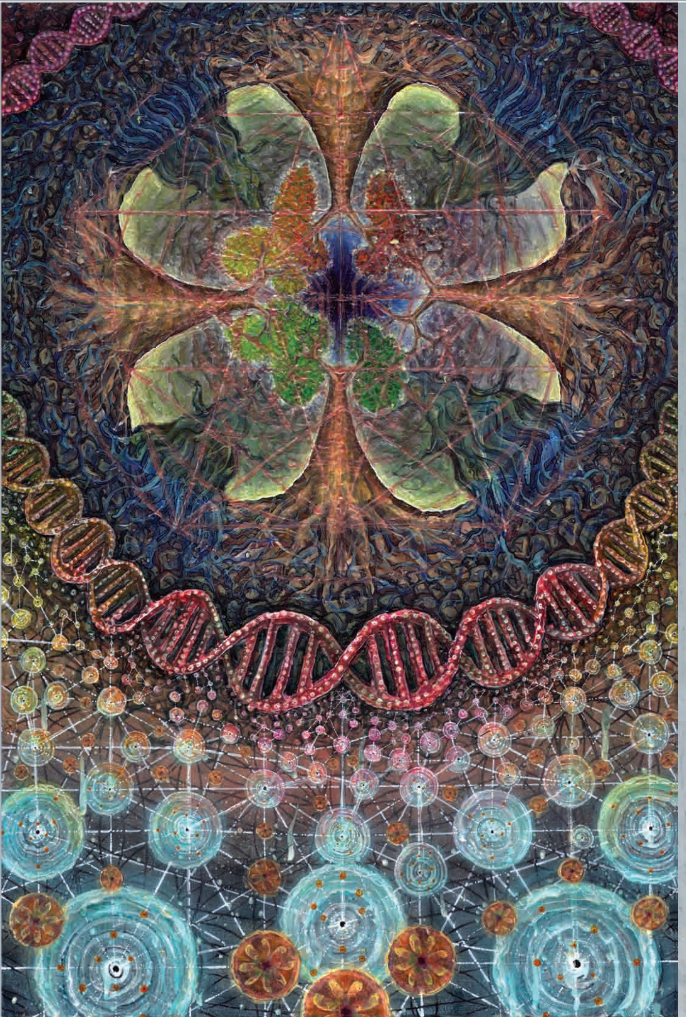
Holoscopic Nature
