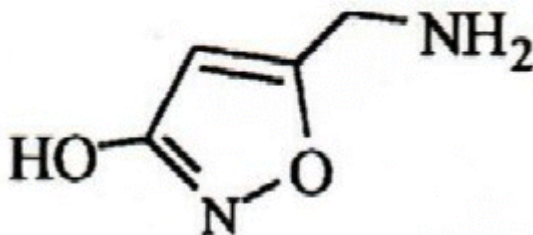
Muscimol
