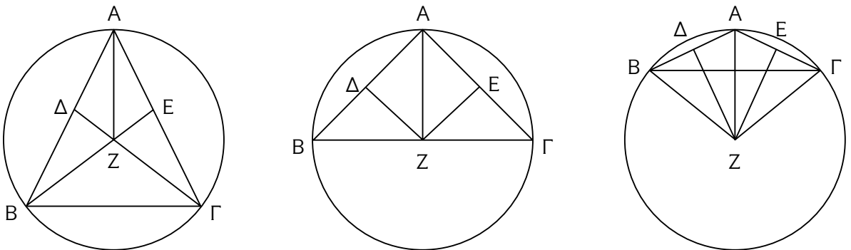
Figure 5.8. Euclid’s Elements IV.5.
