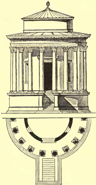
FIG. 52.—CIRCULAR TEMPLE. TIVOLI.
