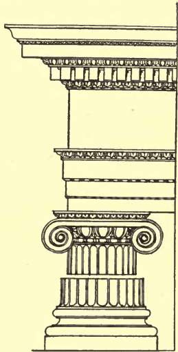
FIG. 43.—ROMAN IONIC ORDER.
