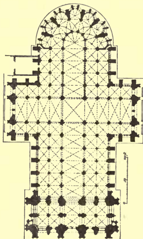
FIG. 146.—COLOGNE CATHEDRAL. PLAN.
