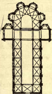
FIG. 98.—PLAN OF NOTRE DAME DU PORT, CLERMONT.
