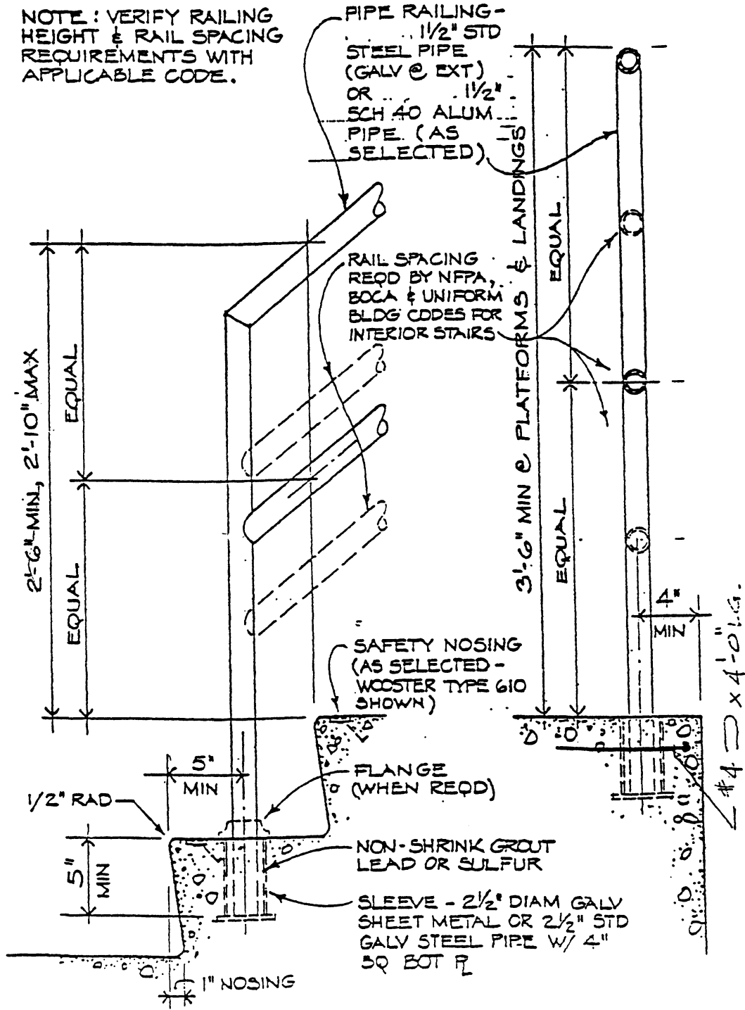
SECTION SCALE: 1 1/2" = 1'-0"
