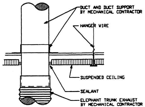
DETAIL ? SCALE: 3"=1'-0" DVG#
