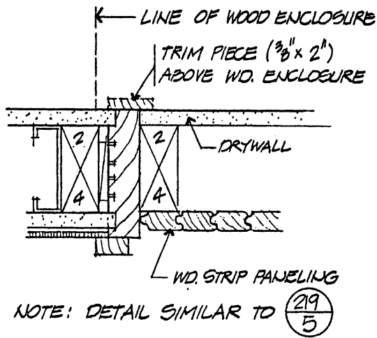
220 JAMB SCALE 3"=1'-0"
