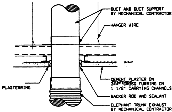
DETAIL ? SCALE: 3"=1'-0" DVG#
