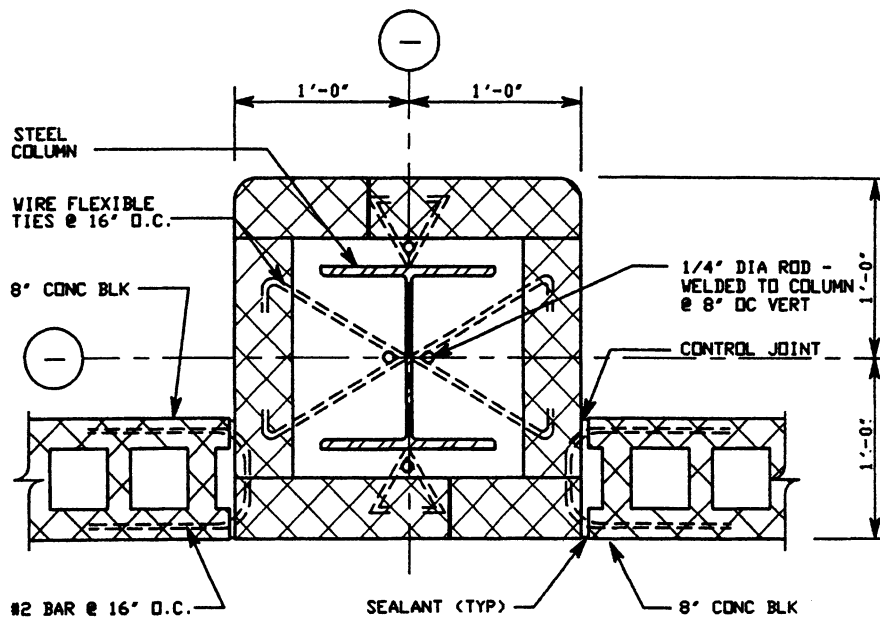
DETAIL SCALE: 1 1/2" = 1'-0"
