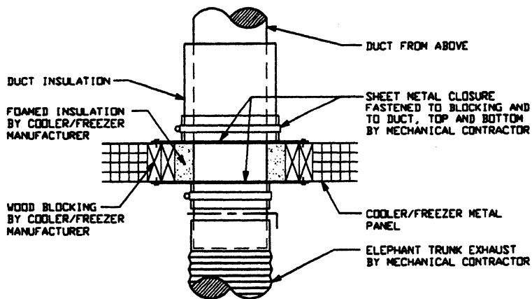
DETAIL ? SCALE: 3"=1'-0" DVG#
