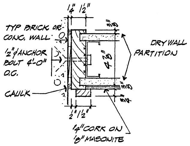
221 JAMB
