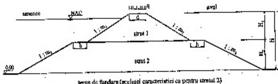
Figura 1.1. Dig de pământ
