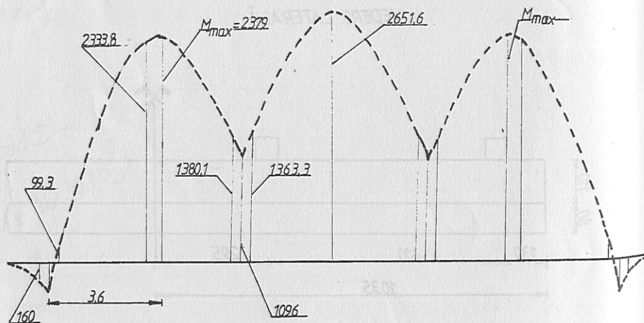
DIAGRAMA DE MOMENT PRIN METODA WINKLER
