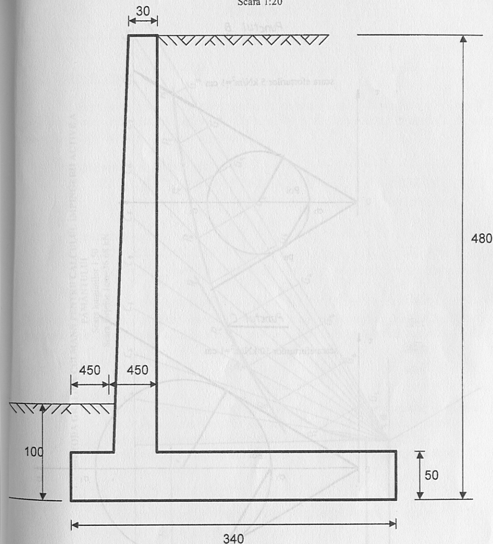
SECȚIUNE TRANSVERSALĂ Scara 1:20
