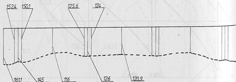
DIAGRAMA DE PRESIUNE PRIN METODA WINKLER
