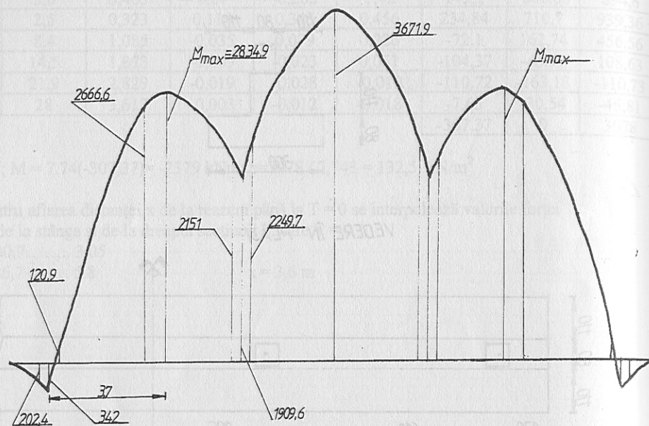
DIAGRAMA DE MOMENT PRIN METODA WINKLER
