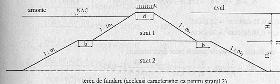
Figura A.1. Dig de pământ
