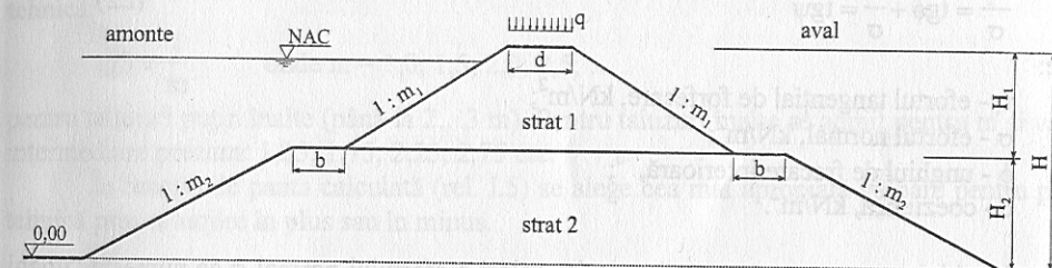
Figura I.1. Dig de pământ
