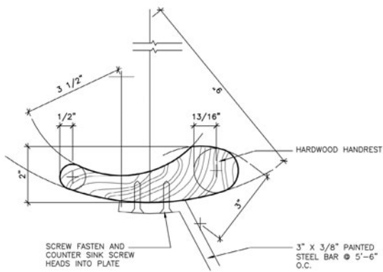
6 guardrail #2 handrest scale: 6"=1'-0"
