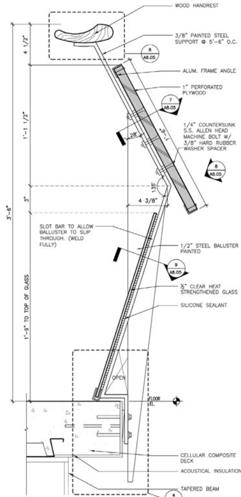
5 guardrail #2 scale: 3"=1'-0"
