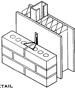
ADJUSTABLE UNIT TIES—STUD
