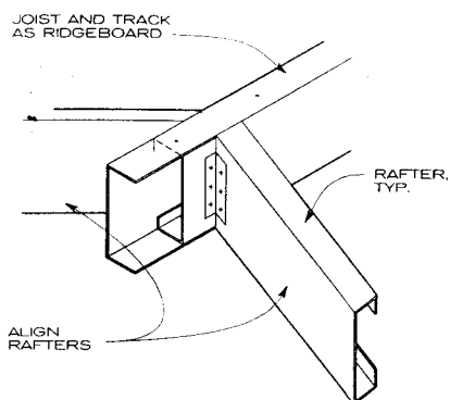
RIDGEBOARD
