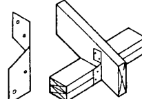
TY-DOWN ANCHOR
