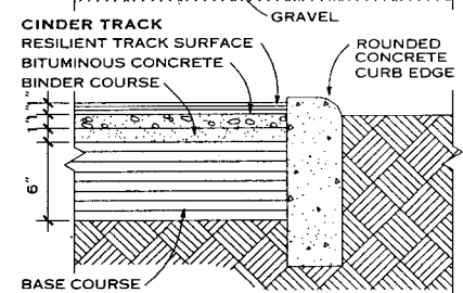
EDGE CONDITIONS
