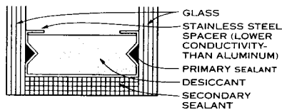
WARM EDGE SPACER
