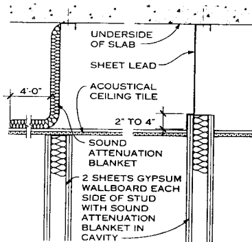
PLENUM BARRIERS
