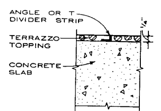
THIN-SET TERRAZZO
