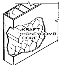
FLUSH DOOR CORE
