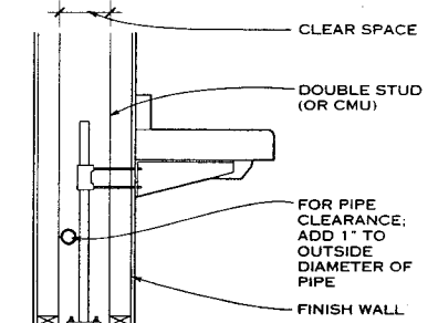
DOUBLE STUD OR CMU
