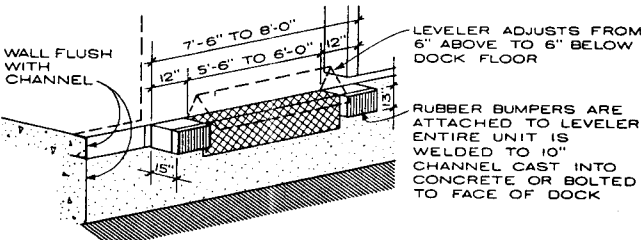
EDGE OF DOCK LEVELER
