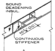
FLUSH CONSTR.
