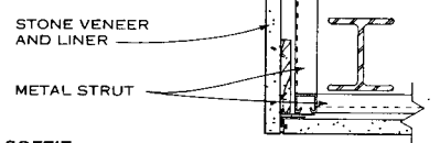
SOFFIT
