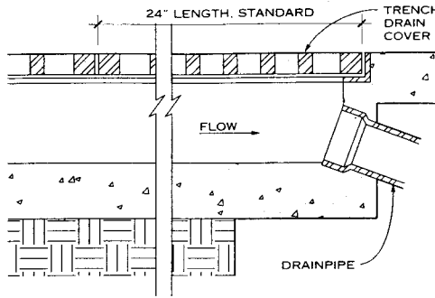
LONGITUDINAL SECTION
